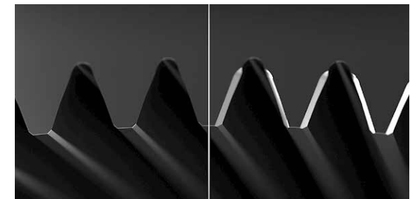
左侧未使用VarioChamfer工艺去毛刺,右侧使用VarioChamfer工艺去毛刺的比较。
